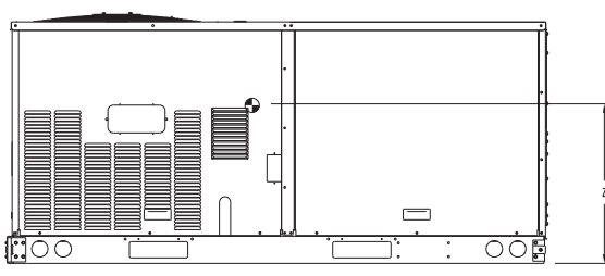
Fig. 3 - Dimensions 50TC-A07
